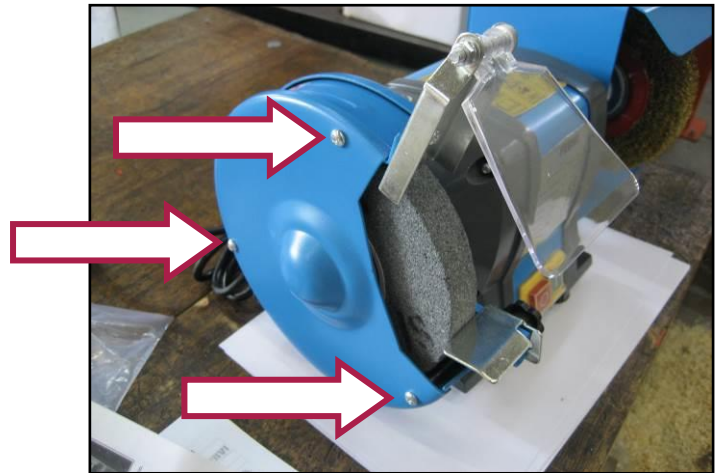
Figura 13 – Carter di protezione.
