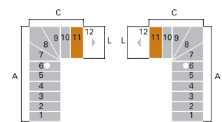
vista frontale con 2 lati di ringhiera
