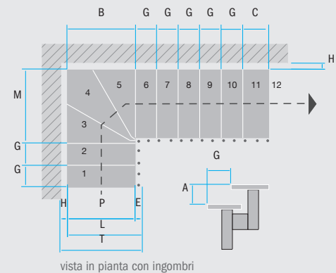
vista in pianta con ingombri
