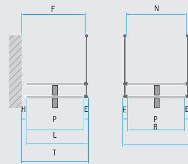
vista frontale con 1 lato di ringhiera
